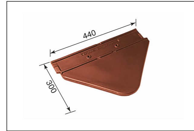
Подконьковая черепица
