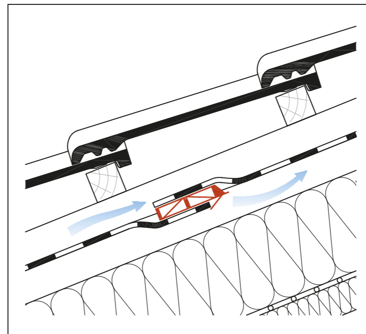
Рисунок 17.4 – Вентиляционный элемент
