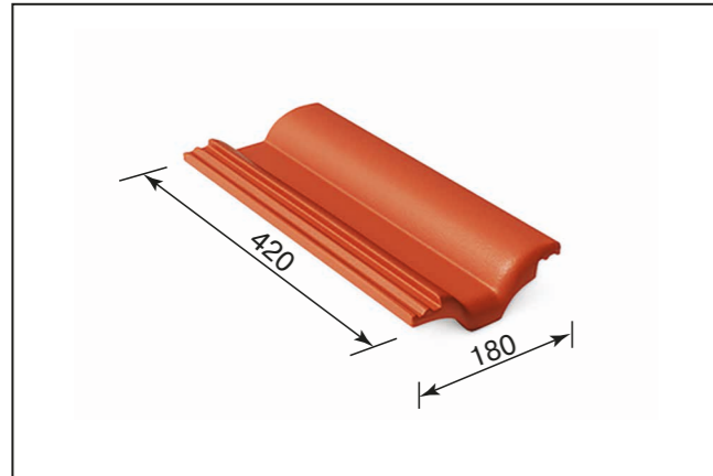
Половинчатая черепица
