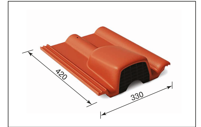
Вентиляционная черепица
