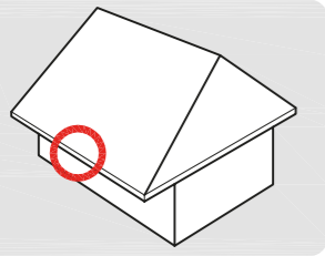
Узел 8 Карнизный свес. Утепленная крыша. Кровли с рекомендуемыми и малыми уклонами, со сплошным настилом, с двумя вентиляционными каналами.
