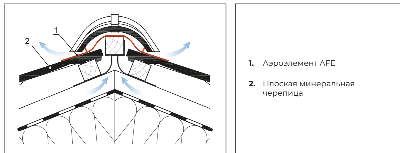
Рисунок 10.2 – Обустройство конька с применением аэроэлемента AFE и плоской минеральной черепицы
