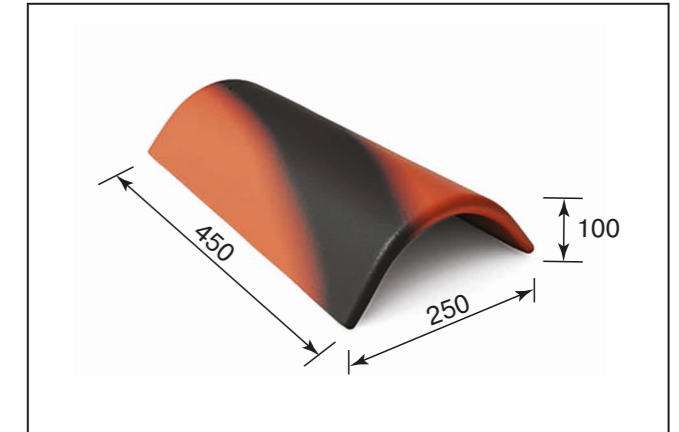
Коньковая черепица
