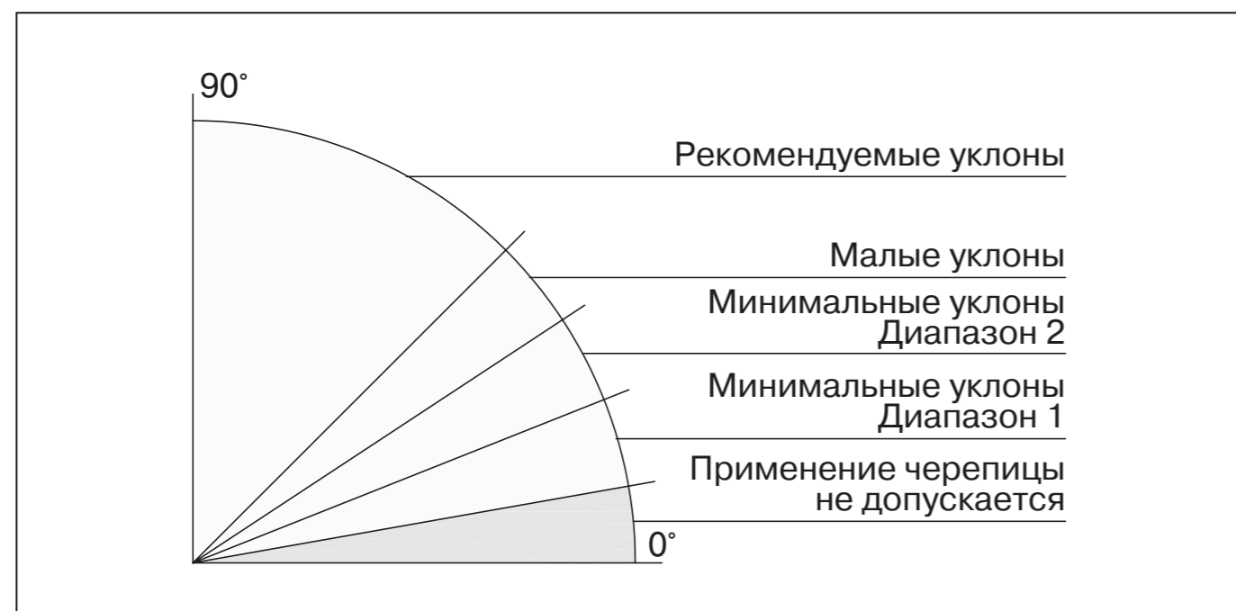
Рисунок 2.1 – Виды уклонов
