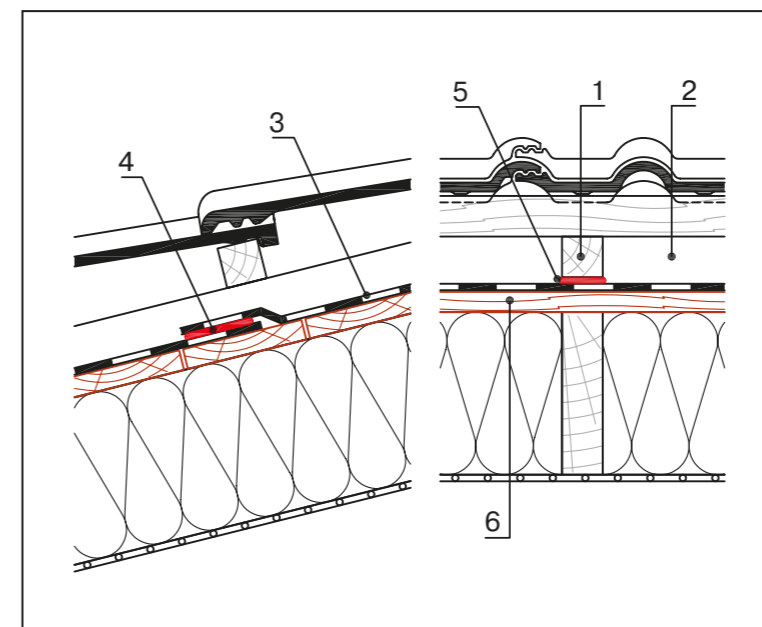
Рисунок 7.5 – Кровля с минимальным уклоном (Диапазон 2), с одним вентиляционным каналом
