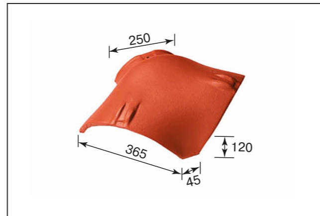
Вальмовая черепица (Кониш HO)
