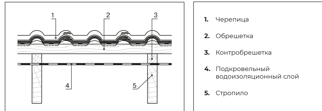
Рисунок 3.1 – Кровля неутепленной крыши
