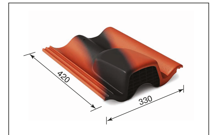
Вентиляционная черепица
