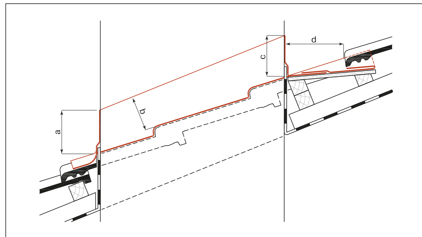
Рисунок 16.2 – Схема примыкания
