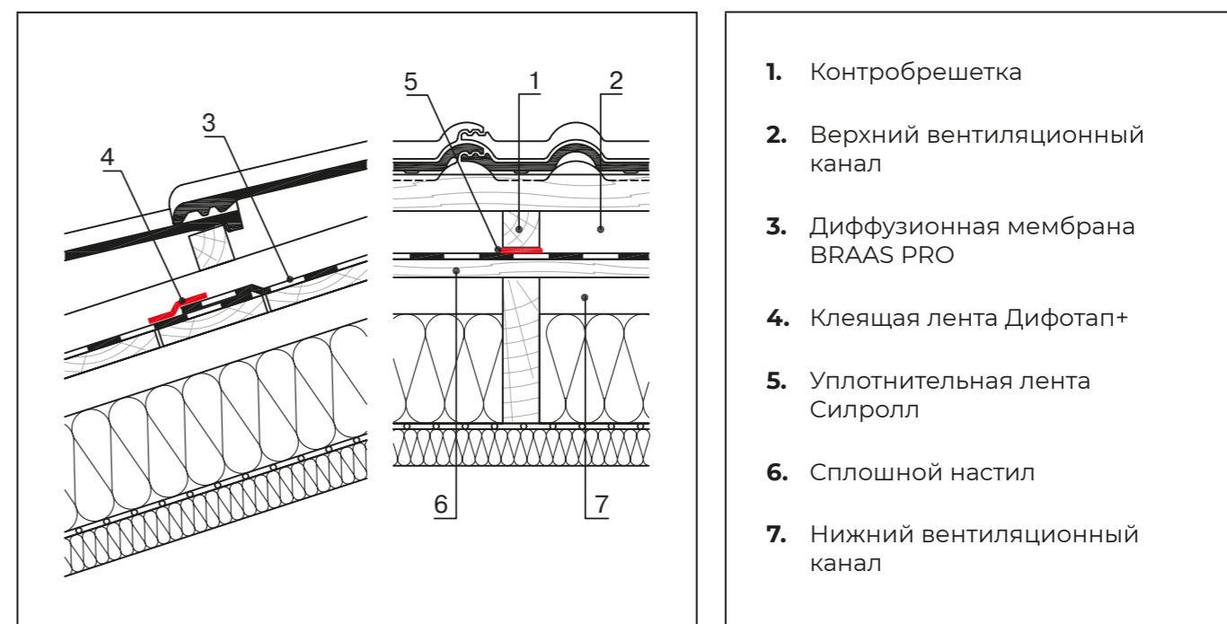
Рисунок 7.4 – Кровля с малым уклоном, со сплошным настилом, с двумя вентиляционными каналами
