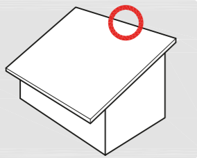
Узел 22 Конек с применением коньковой черепицы. Односкатная утепленная крыша. Кровли с рекомендуемыми и малыми уклонами.
