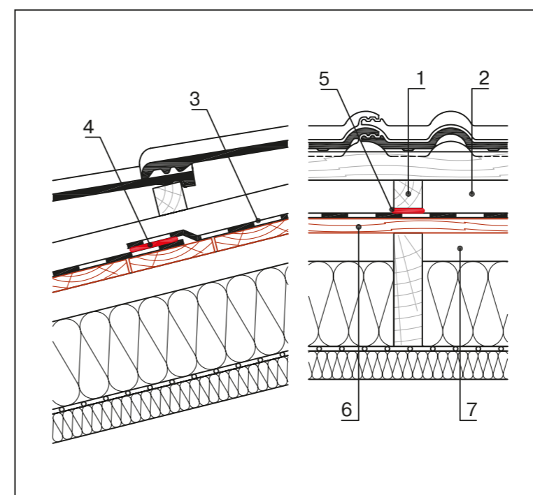
Рисунок 7.6 – Кровля с минимальным уклоном (Диапазон 2), с двумя вентиляционными каналами
